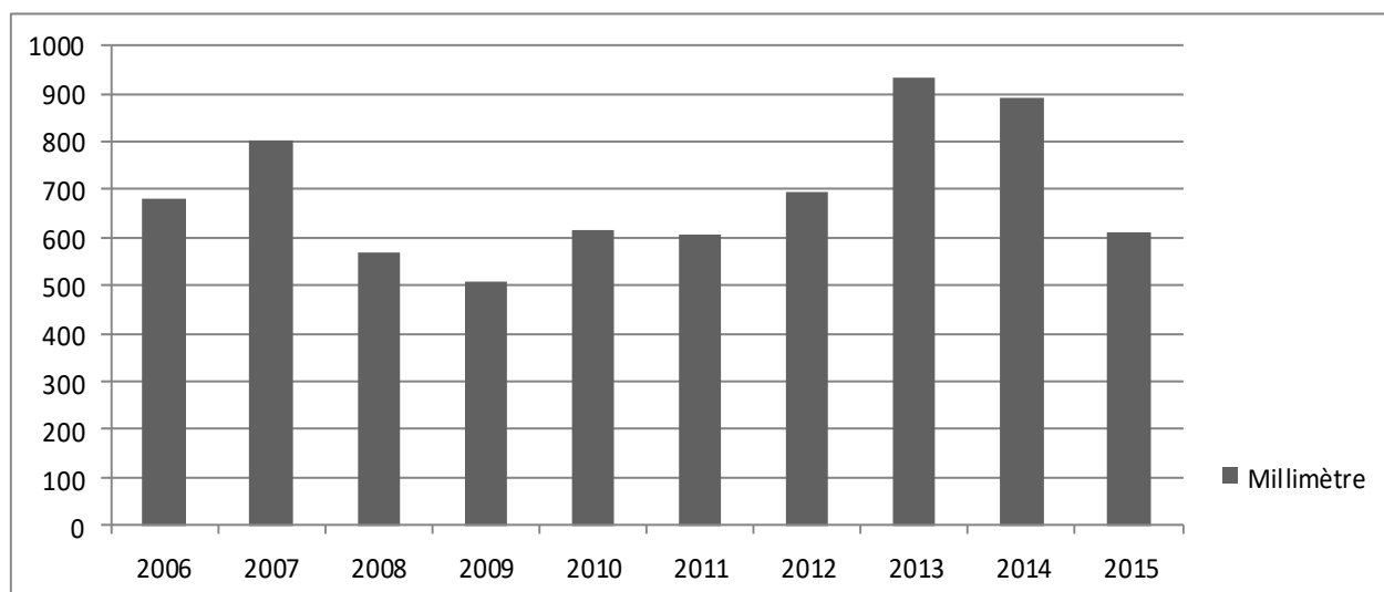
Evolution de la pluviométrie de 2006 à 2015 en Mm
